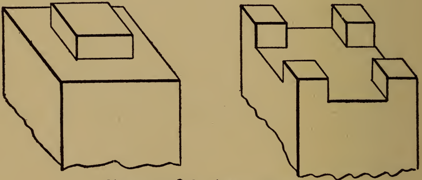
Fig. 293. Spur Tenon.
