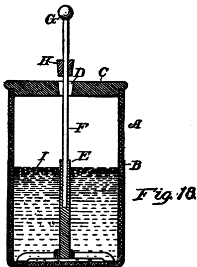
LEYDEN JAR
